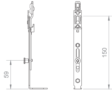
Bottom Extension Se 180°
