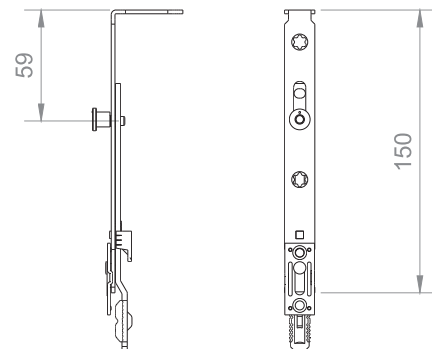
Bottom Extension Se 90°
