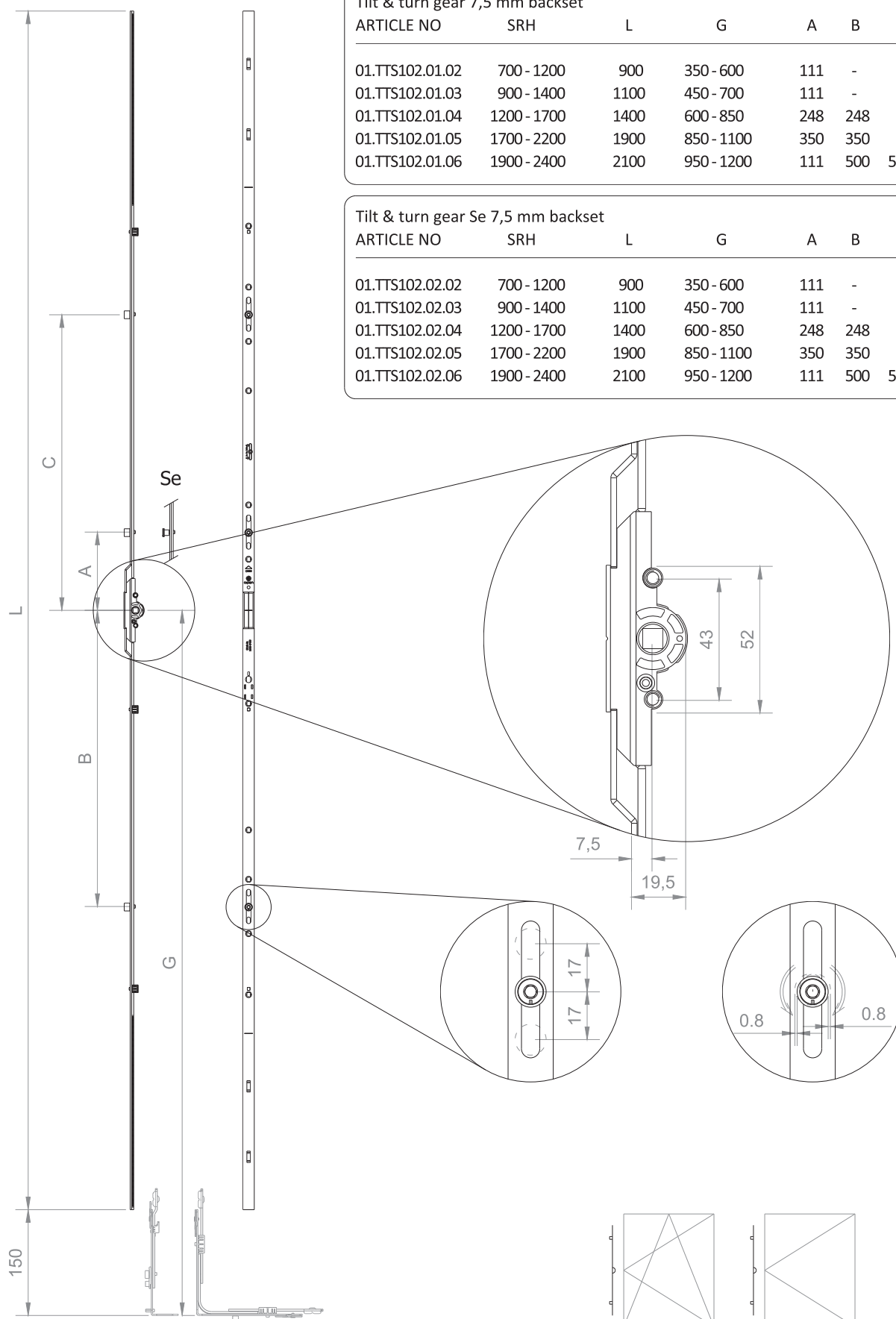
Tilt & turn gear 7,5 mm backset
