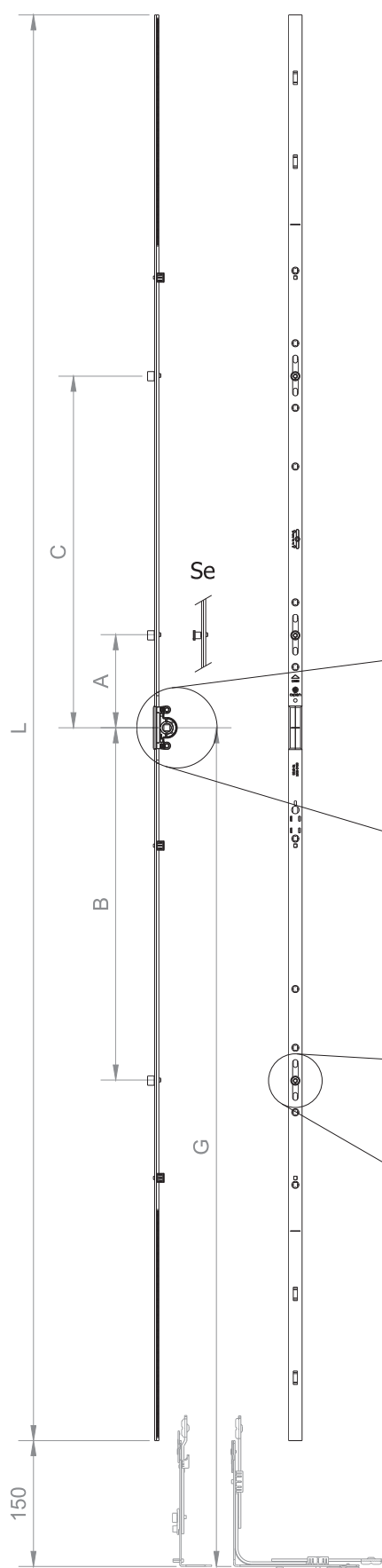
Tilt & turn gear Se 15 mm backset
